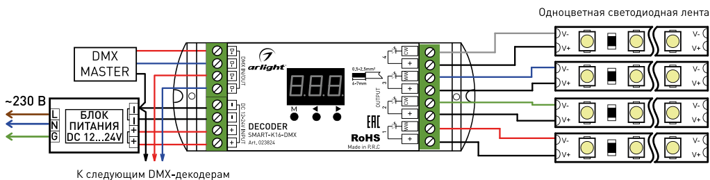
Рис. 1. Общая схема подключения декодера.
